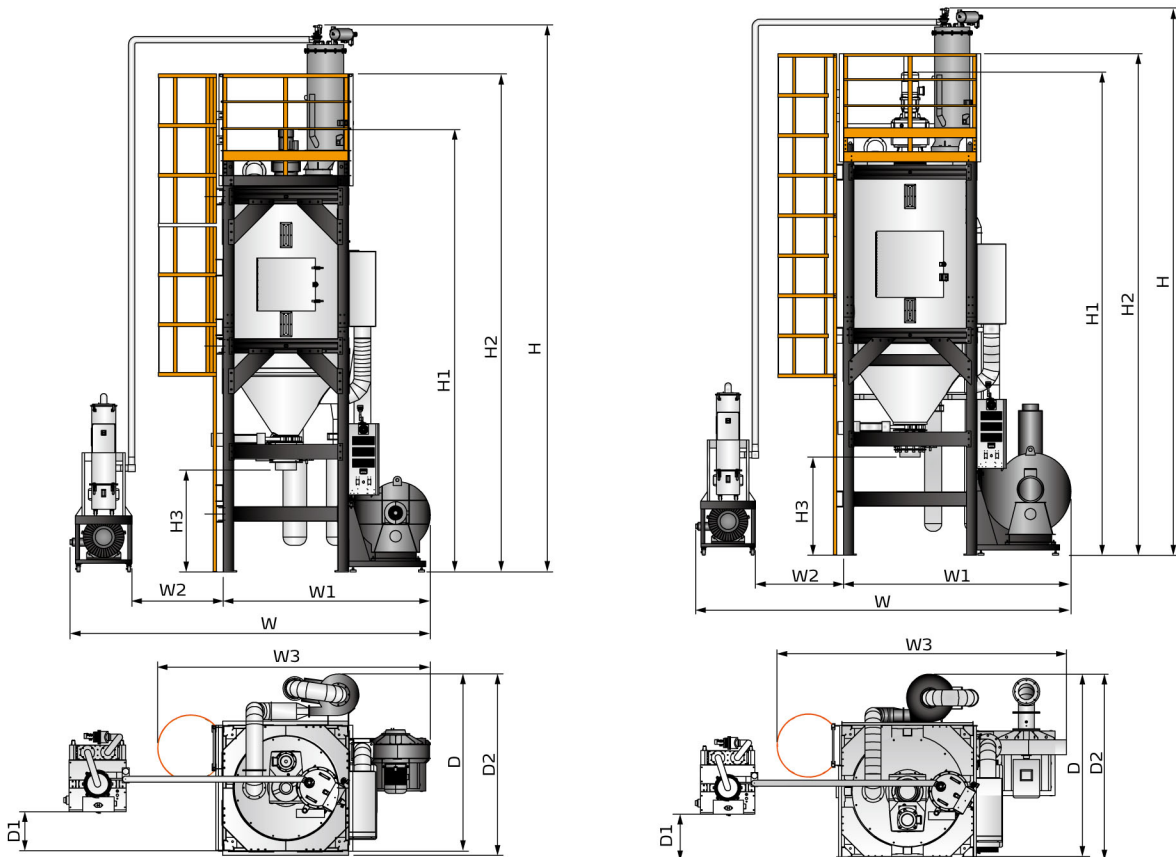
SICR-1600U(选装护梯)
