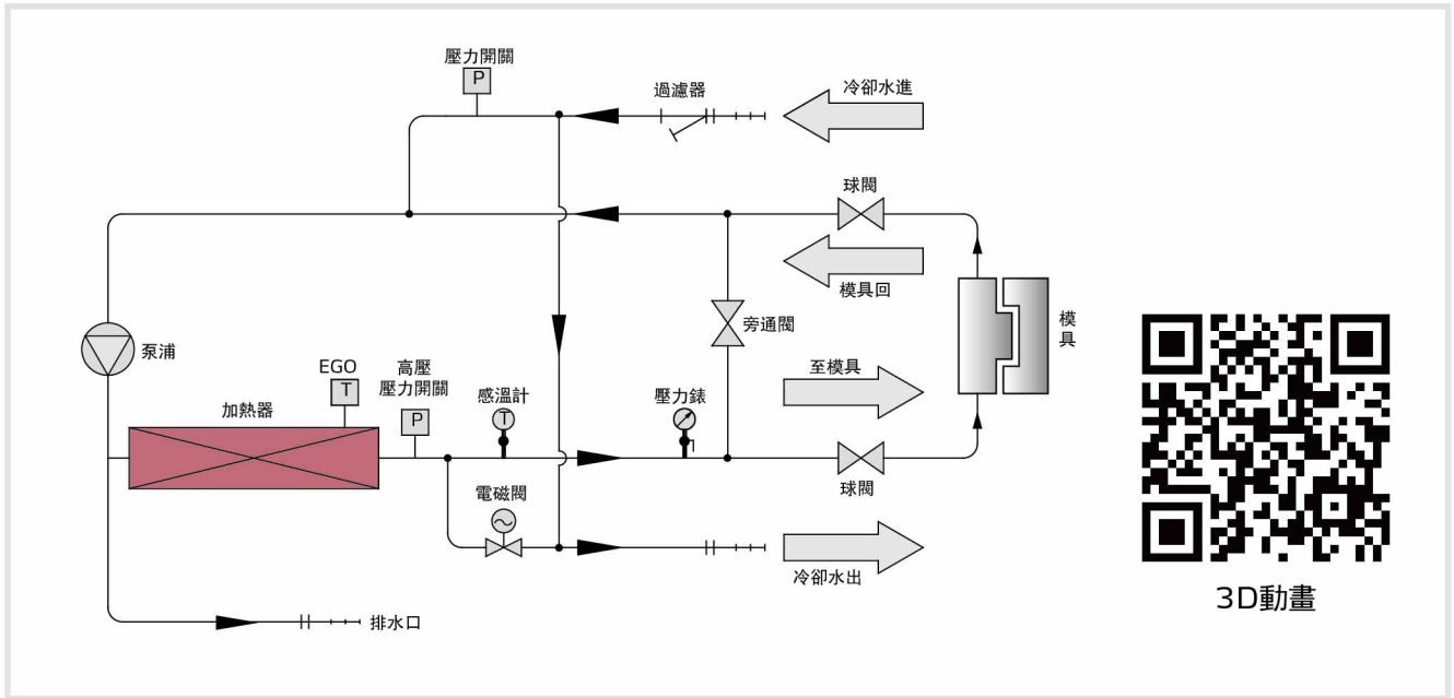
STM-W標準型工作原理圖 (直接冷卻)
