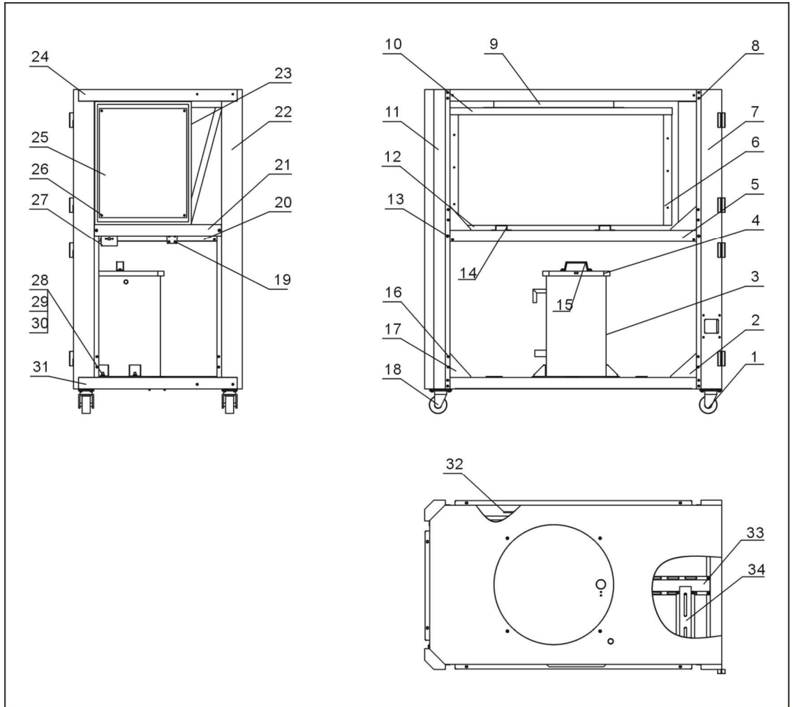
图 2-7：机架图(SIC-12A-R2)
