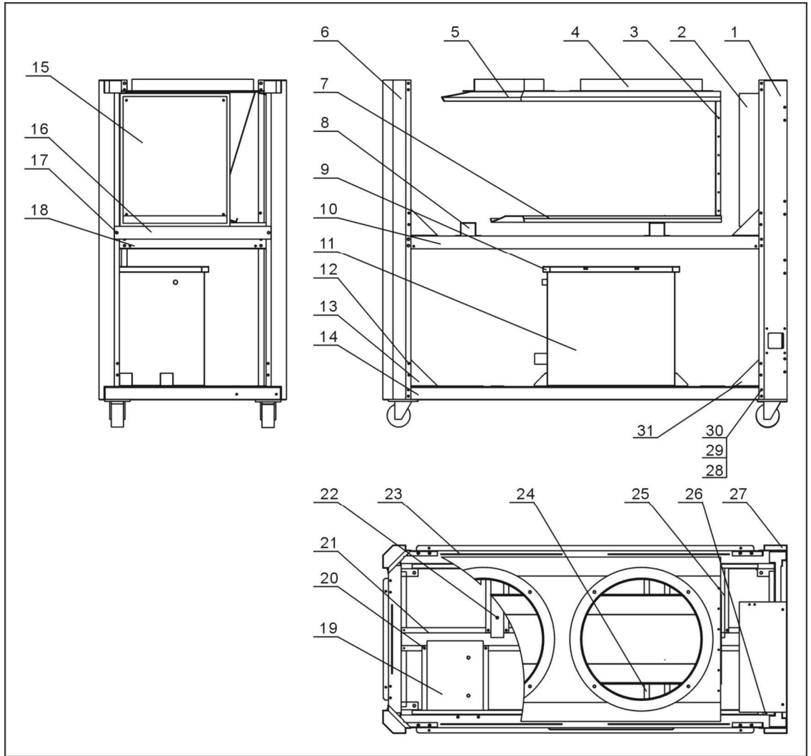
图 2-11：机架图(SIC-18A-R2~24A-R2)
