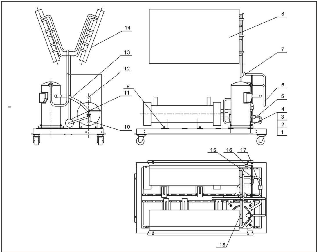
图 2-5：冷媒系统图(SIC-7.5A-R2)
