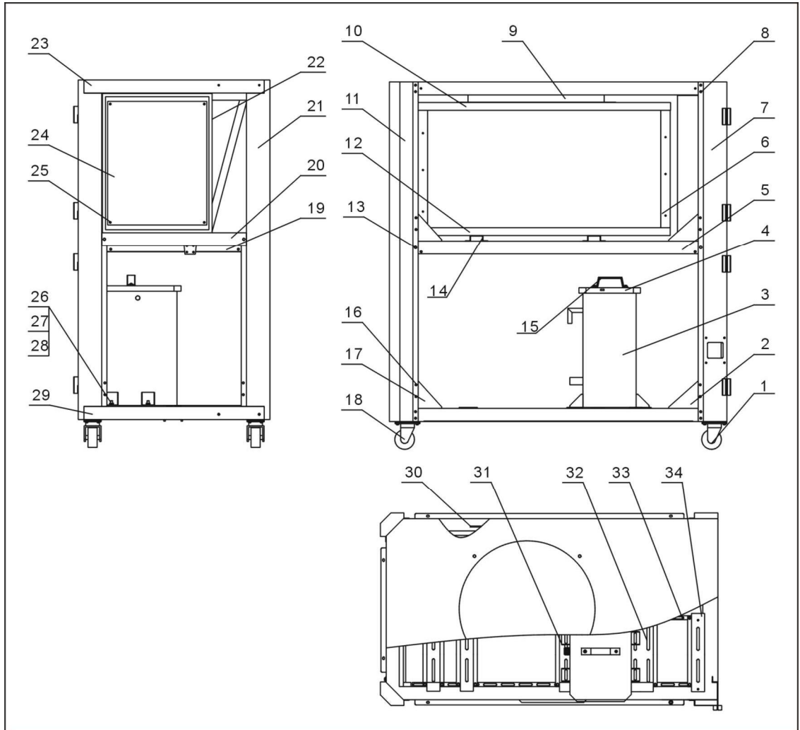
图 2-3: 机架图(SIC-7.5A-R2)
