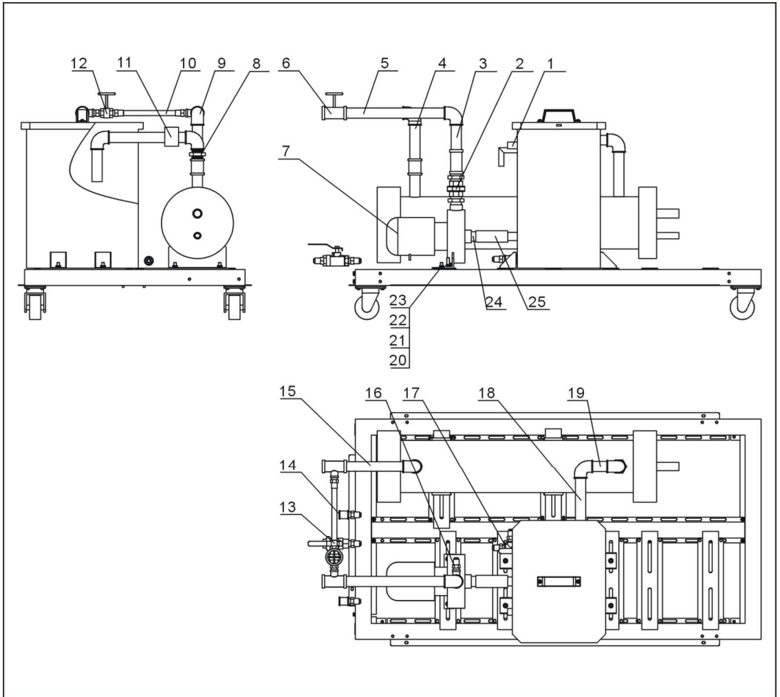
图 2-8: 水系统图(SIC-12A-R2)
