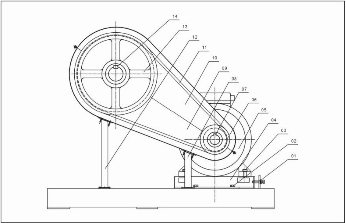
图 2-10: 传动件图
