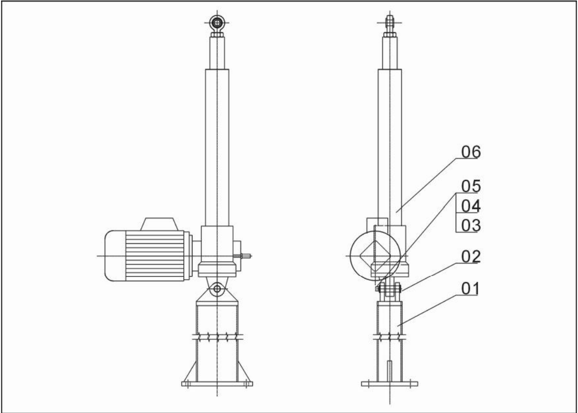
图 2-17: 电动推杆
