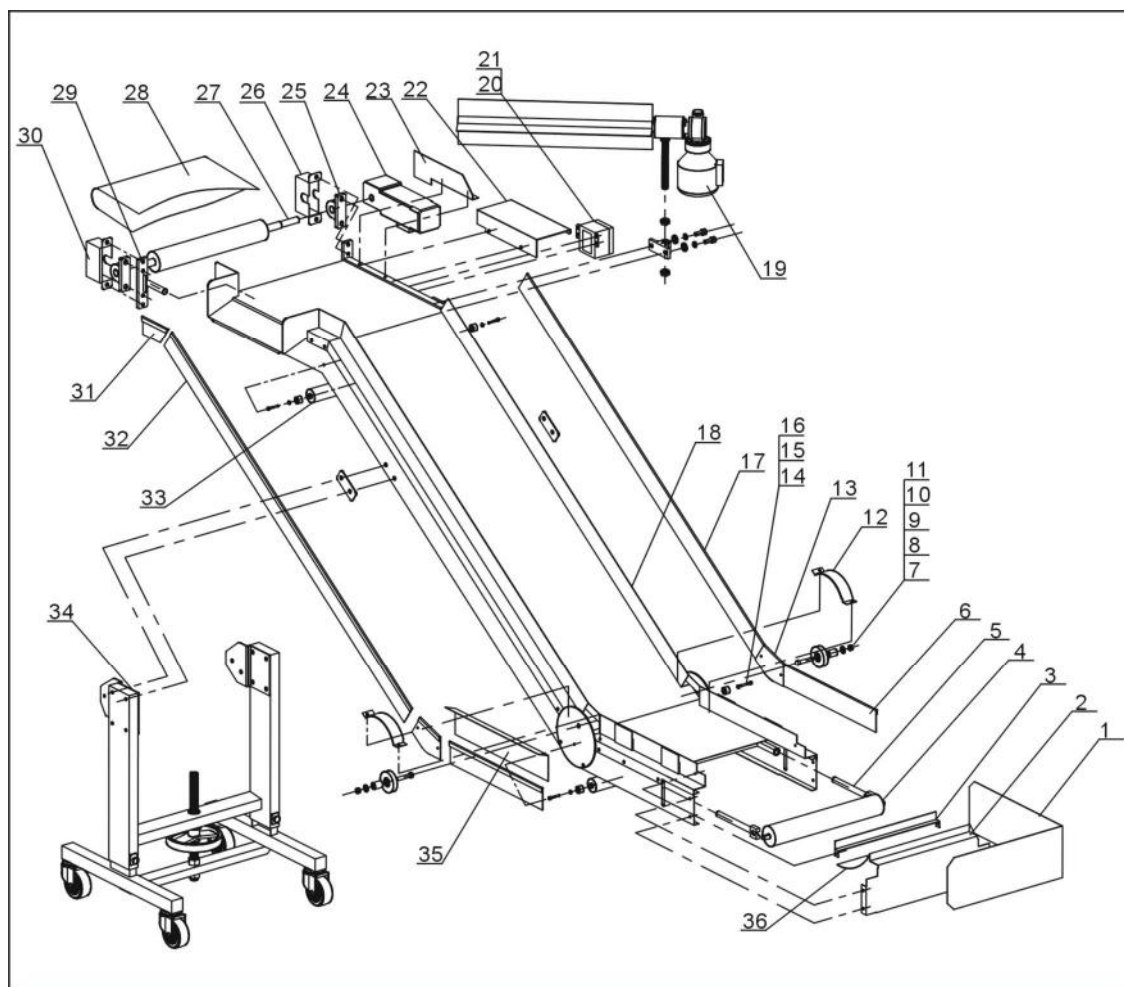
图 2-3：零件图
