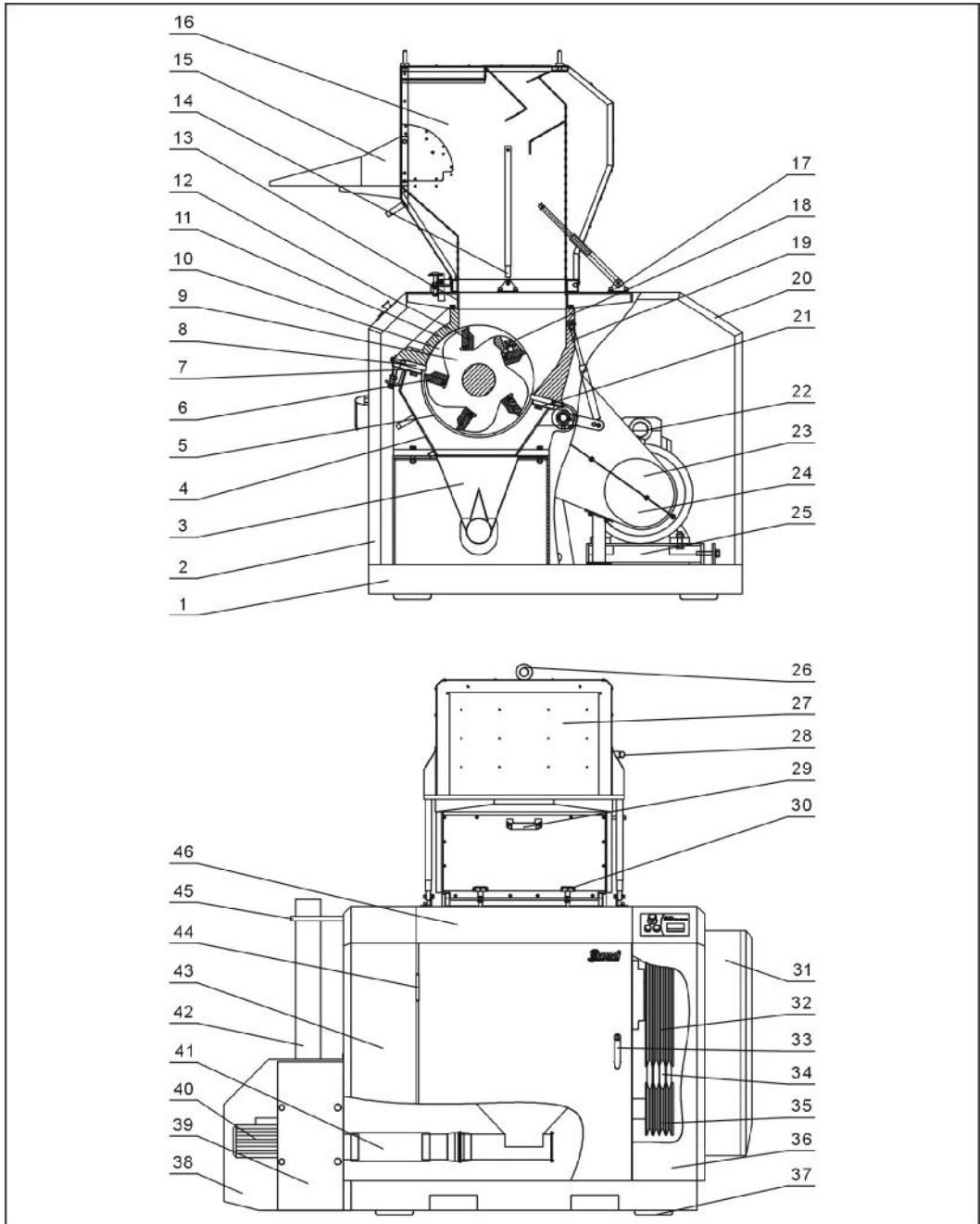
图 2-5：系统结构图
