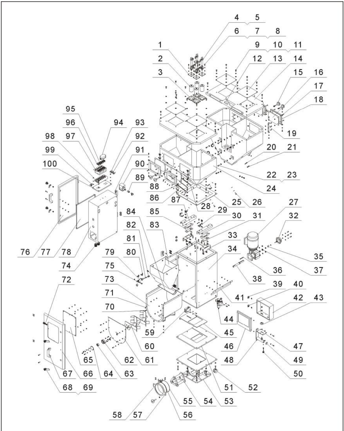
图 2-8: SGB-600-4 零件图
