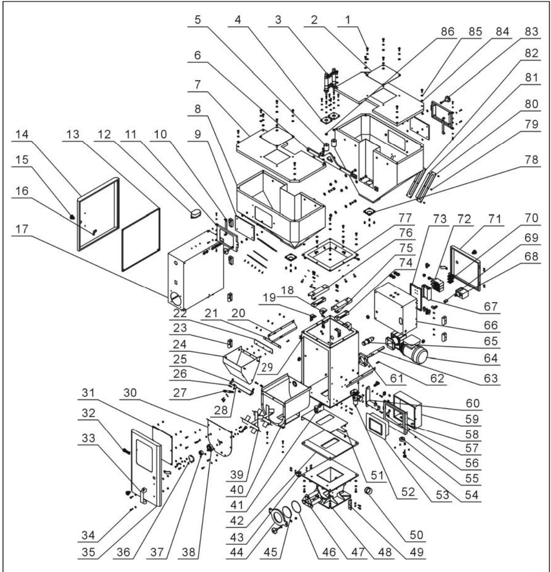
图 2-3: SGB-200-2 零件图
