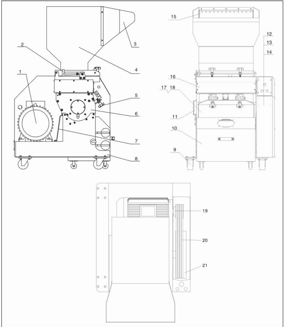
图 2-5: 系统结构图(SG-23E / 30E)
