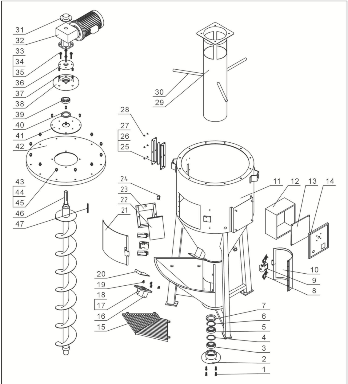
图 2-2: 零件图(SVM-160U/300U)
