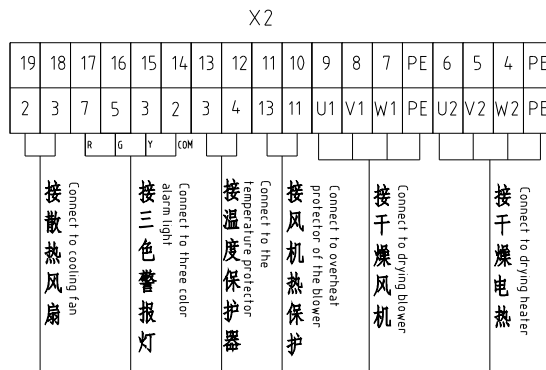
电控箱内部 Inside the electric control box
