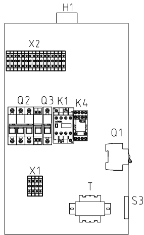
电控箱内部 Inside the electric control box
