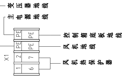
控制箱电器安装板
