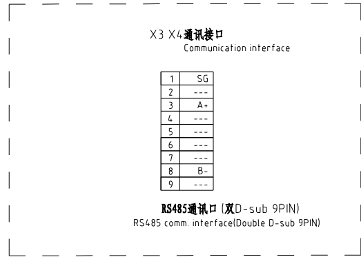
RS485 通讯接线图 RS485 Comm. wiring diagram
