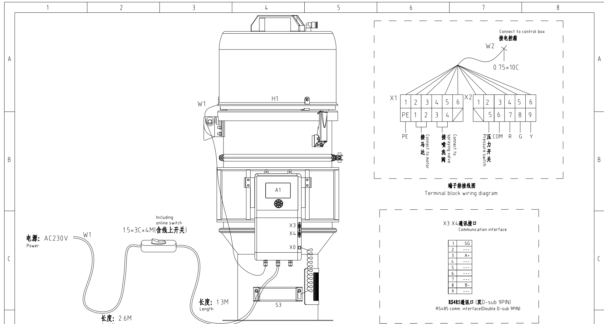
RS485 通讯接线图 RS485 Comm. wiring diagram
