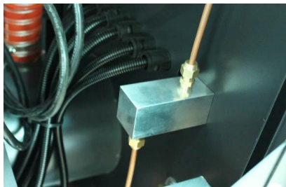
图 2-15: 露点计安装座
