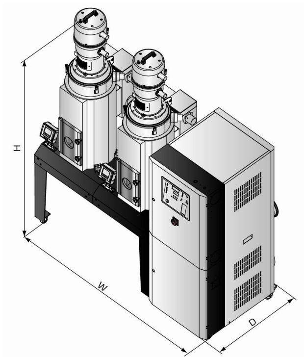
图 1-1: 外形尺寸图
