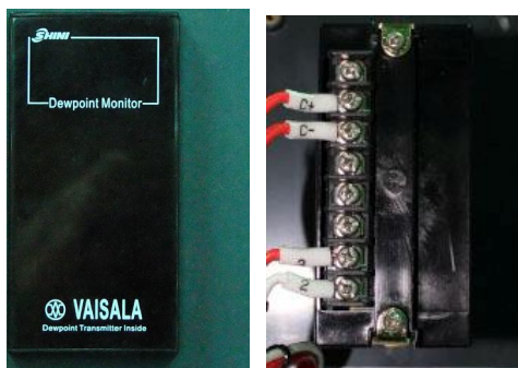
图 2-17: 露点显示器安装
