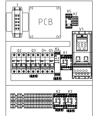
Optional Model Layout 选配机型布局图
