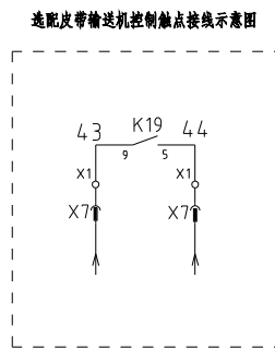
选配皮带输送机控制触点接线示意图
