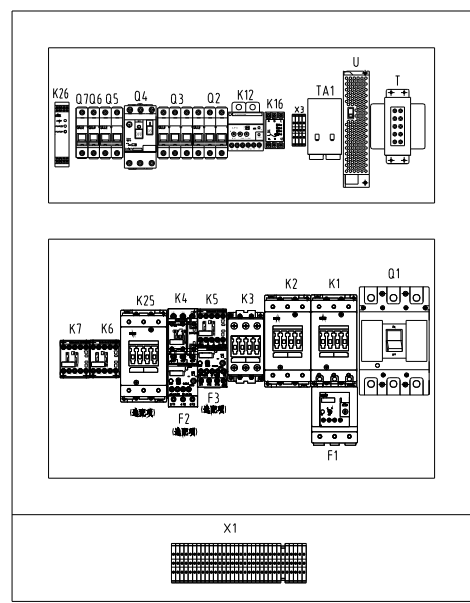
选配机型布局图
