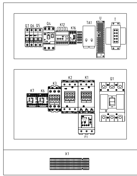
标准机型布局图
