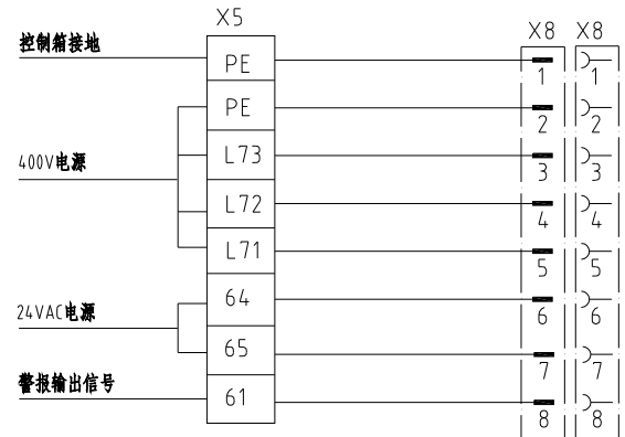
(桶2控制箱内信号)
