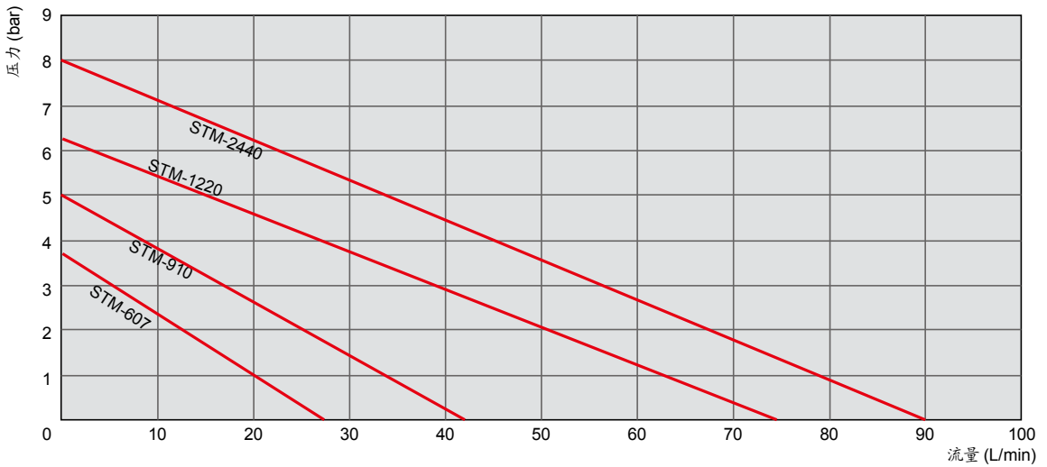
图 1-1: 泵浦曲线图
