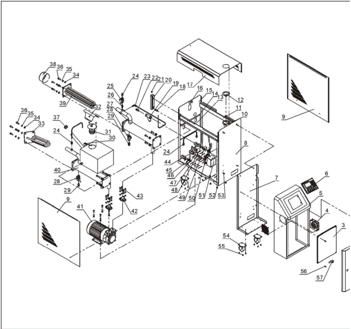
图 2-3: 系统结构图(STM-1220)
