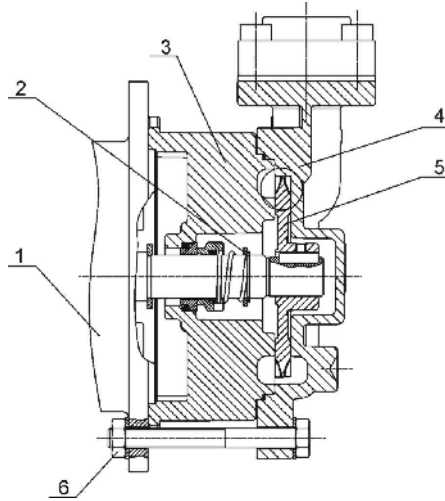
图 2-6: 泵浦图
