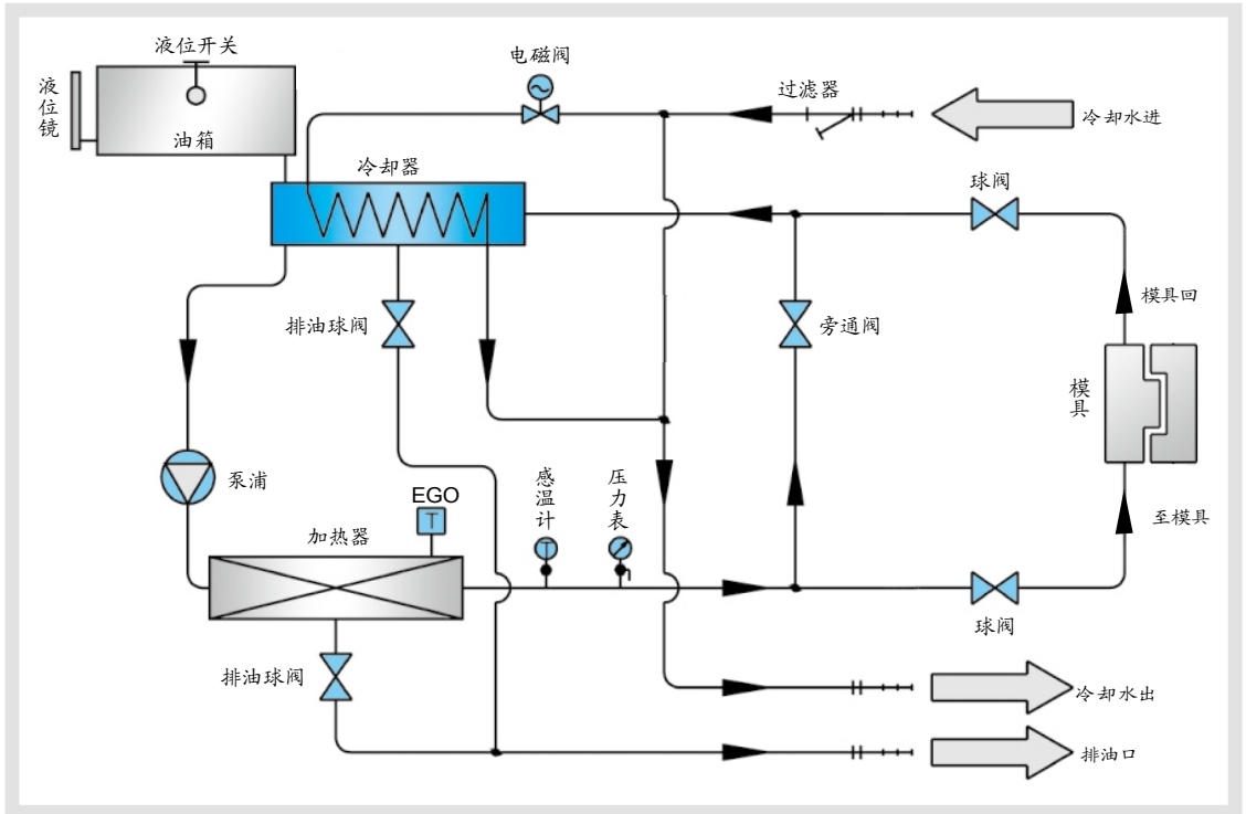
图 2-1: 工作原理图
