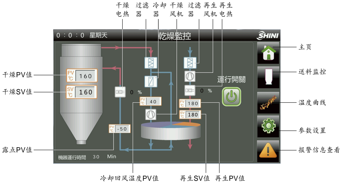
图 4-2：SCD 系列干燥监控画面
