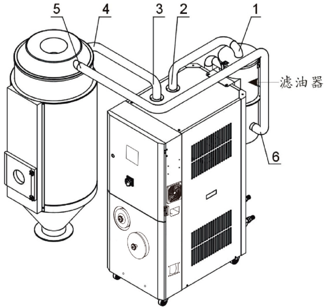
图 3-5: 滤油器安装图
