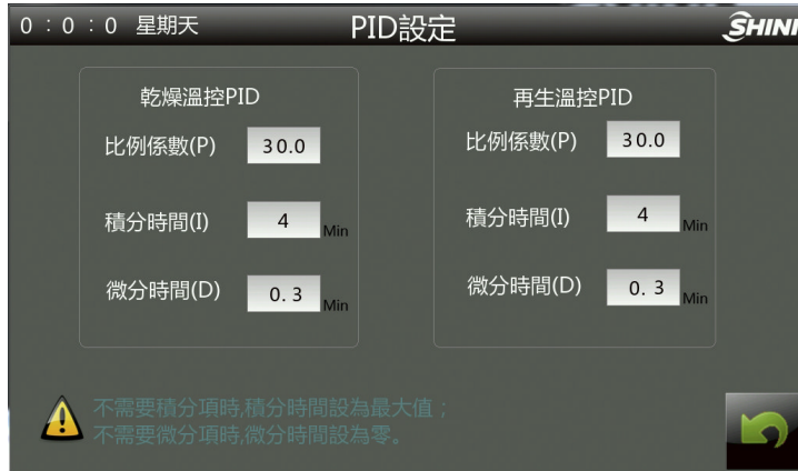
图 4-15: PID 参数设定画面
