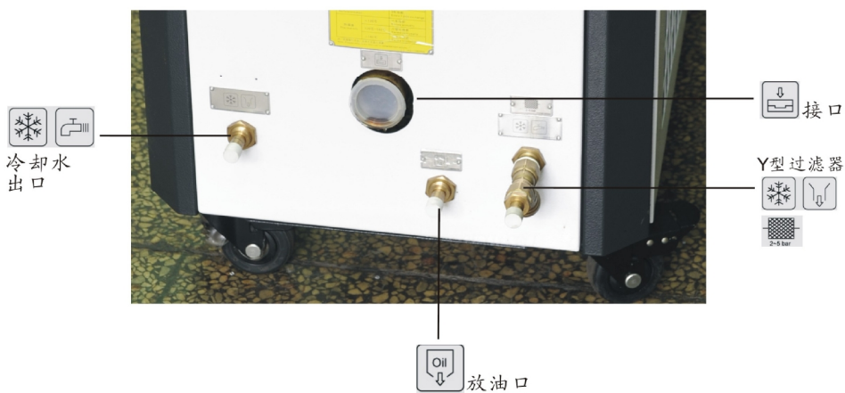
图 3-3：管路的连接
