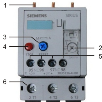
图 2-19：热过载继电器
