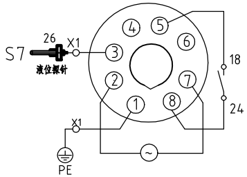
K10 水位继电器1
