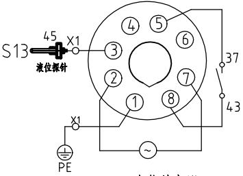
K11 水位继电器2
