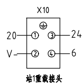
站1重载接头
