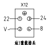
站3重载接头
