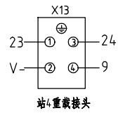
站4重载接头
