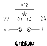
站3重载接头
