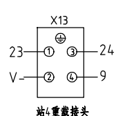
站4重载接头
