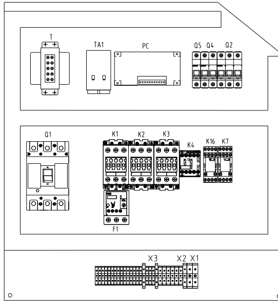
标准机型布局图
