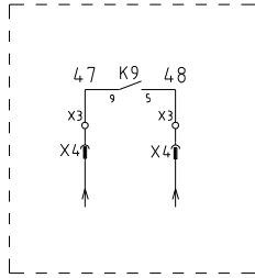
选配皮带输送机控制触点接线示意图
