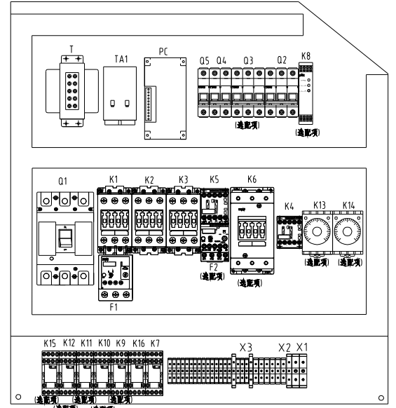
选选项机型布局图
