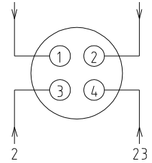
X10金属接头接线示意图 接满料报警装置 (选选项)
