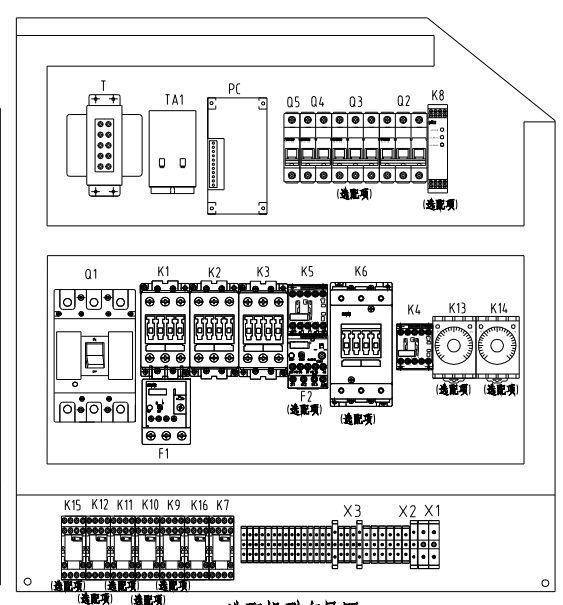
选配机型布局图
