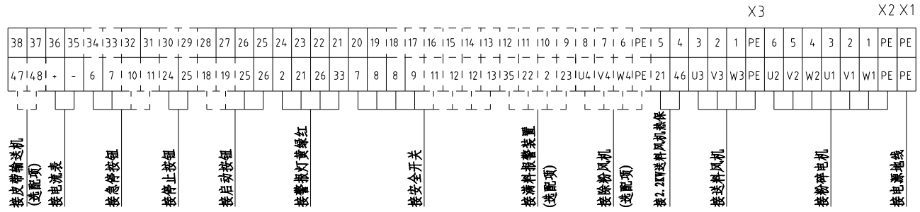
标准机型布局图
