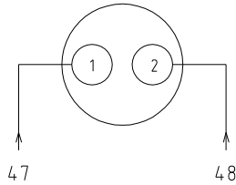
X10金属接头接线示意图 接满料报警装置 (选选项)
