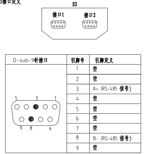
信易RS-485接口定义
