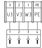
X9 防水接头
