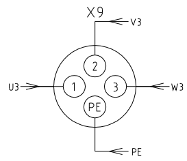
防水接头 (接X8端子)
