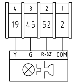
警报灯红黄绿
