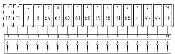
X10 16P 重载接头 (不选配安全继电器时9号改为19号)
