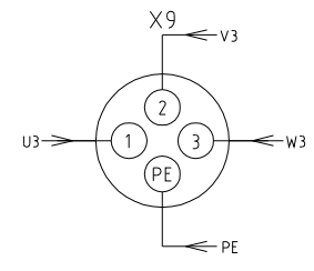
防水接头 (接X8端子)
