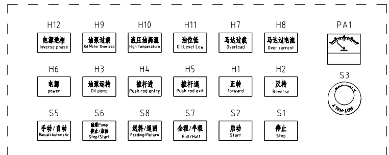
控制面板排布
