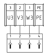
X9 防水接头
