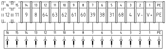
X10 16P 重载接头 (不选安全继电器时9号改为19号)
