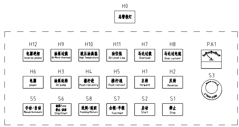
控制面板排布
