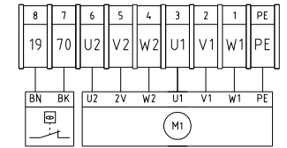
电机热保
