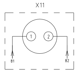
金属接头接线 接皮带输送机 (选选项)
