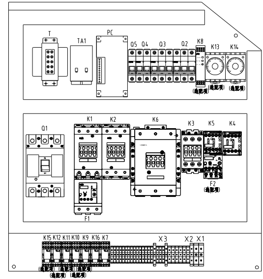
选配机型布局图
