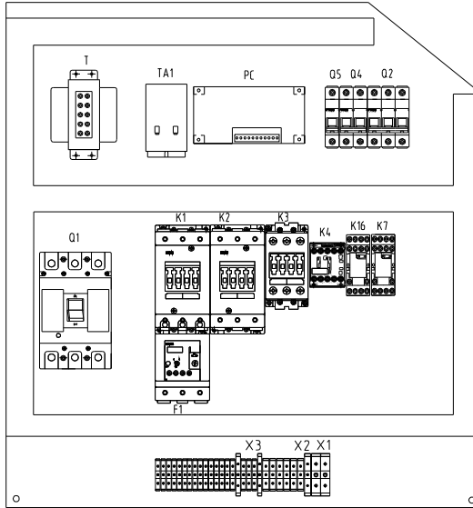
标准机型布局图
