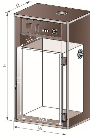
图 1-1: 外形尺寸图
