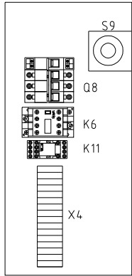
干燥桶1控制箱 Drying hopper 1 Control box
