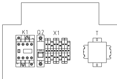
控制箱电器安装板
