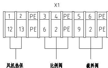
风机热保
