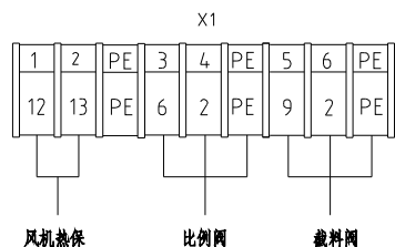
风机热保 比例阀 截料阀
