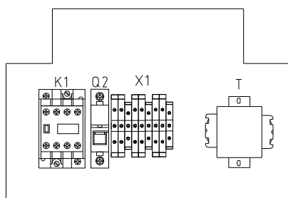
控制箱电器安装板
