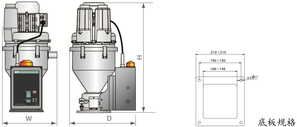
图 1-1: 外形尺寸图
