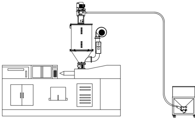
图 5-1：SAL-430/460 安装示意图
