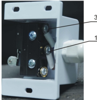
图 4-1：微动开关图
