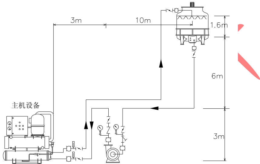
图 9-5：泵浦扬程计算实例图
