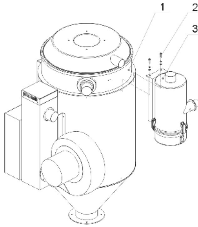
图 2-59: 欧化热风回收安装图
