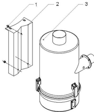
图 2-39: 过滤桶组件安装图
