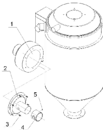
图 2-51: 风车入口法兰安装图
