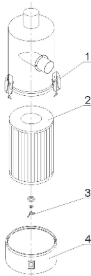
图 2-53: 欧化热风回收器清理图
