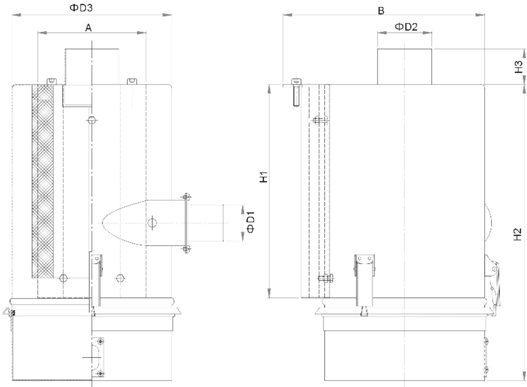
图 2-35: 欧化热风回收器外形尺寸图
