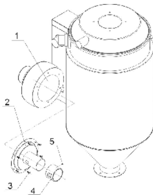
图 2-41: 风车入口法兰安装图
