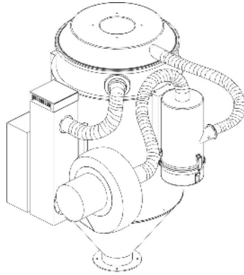
图 2-52: 风管安装图
