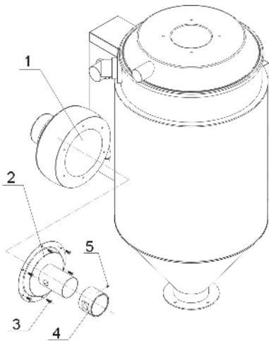
图 2-60: 风车入口法兰安装图
