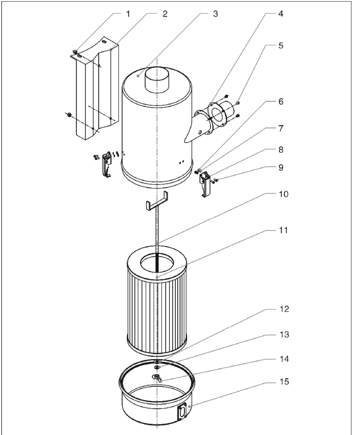
图 2-47: 欧化热风回收器分解图
