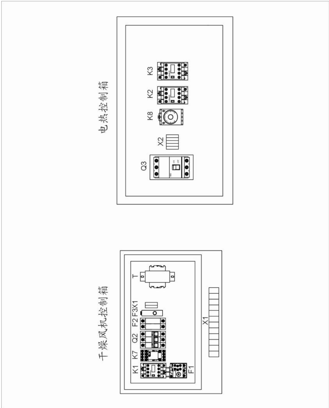
图 2-15: 电气元件布置图(SHD-1500U~2000U)
