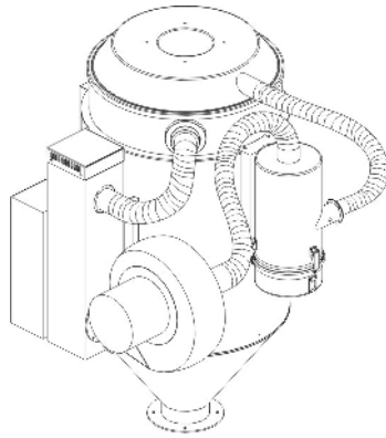
图 2-42: 风管安装图
