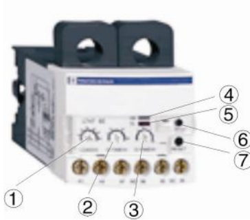
图 2-31: 电流继电器
