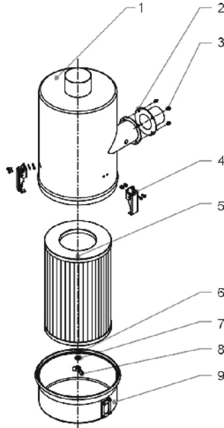
图 2-57: 过滤器及集尘桶安装图
