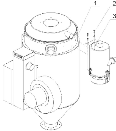
图 2-40: 欧化热风回收器安装图
