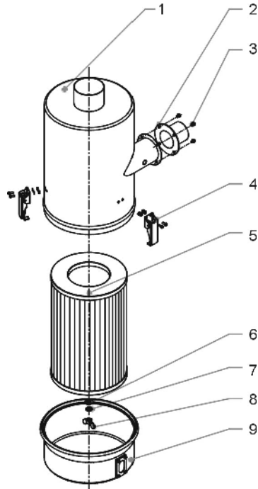
图 2-38: 过滤器及集尘桶安装图
