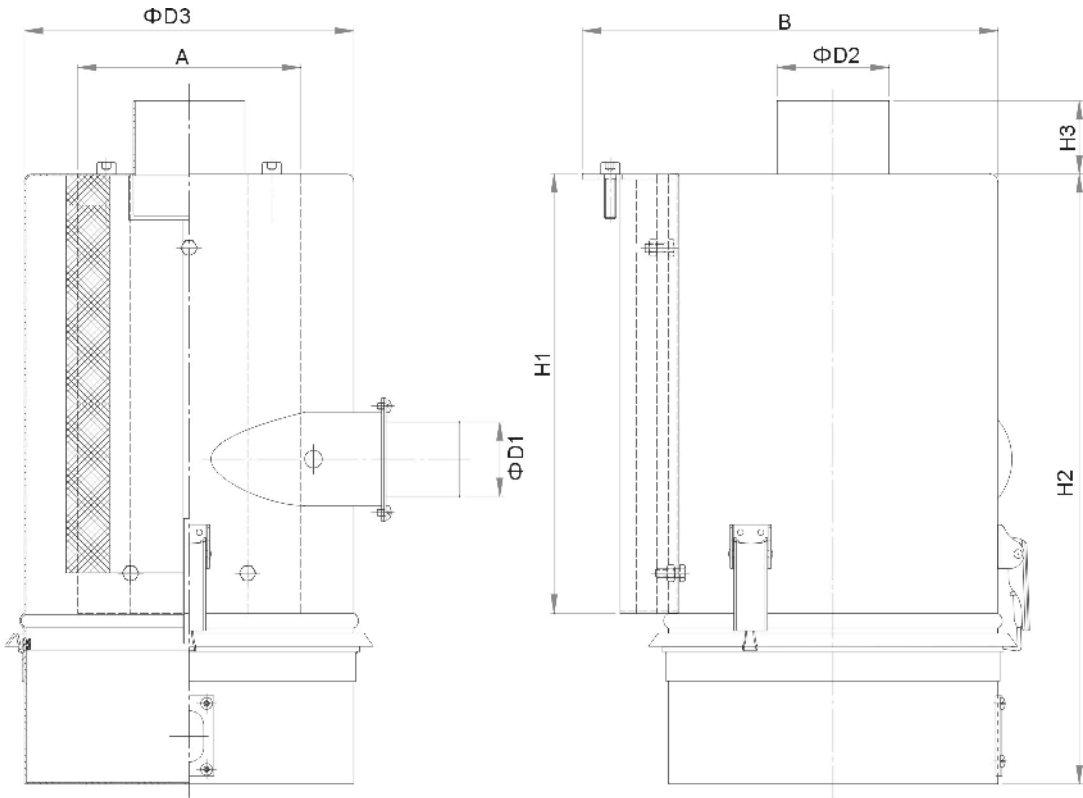
图 2-55: 欧化空气滤清器外形尺寸图
