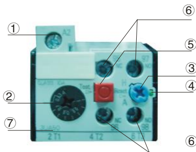
图 2-30: 热过载继电器
