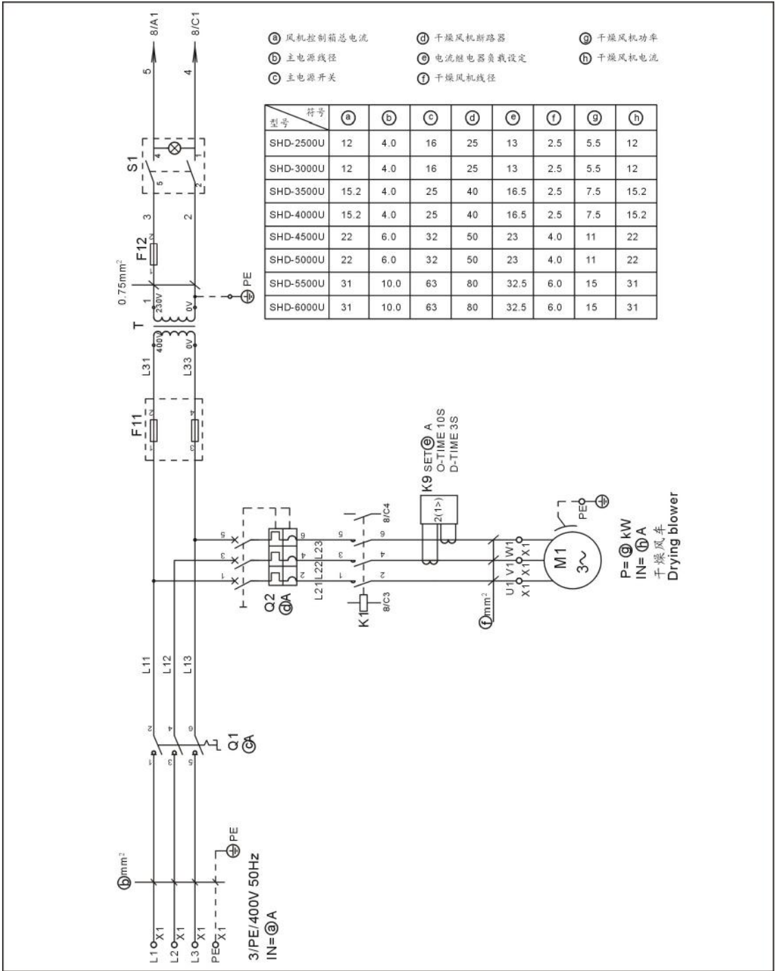
图 2-16: 主电路图一(SHD-2500U~6000U 400V)
