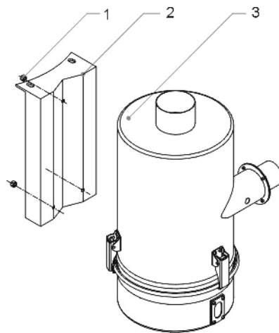
图 2-49: 过滤桶组件安装图
