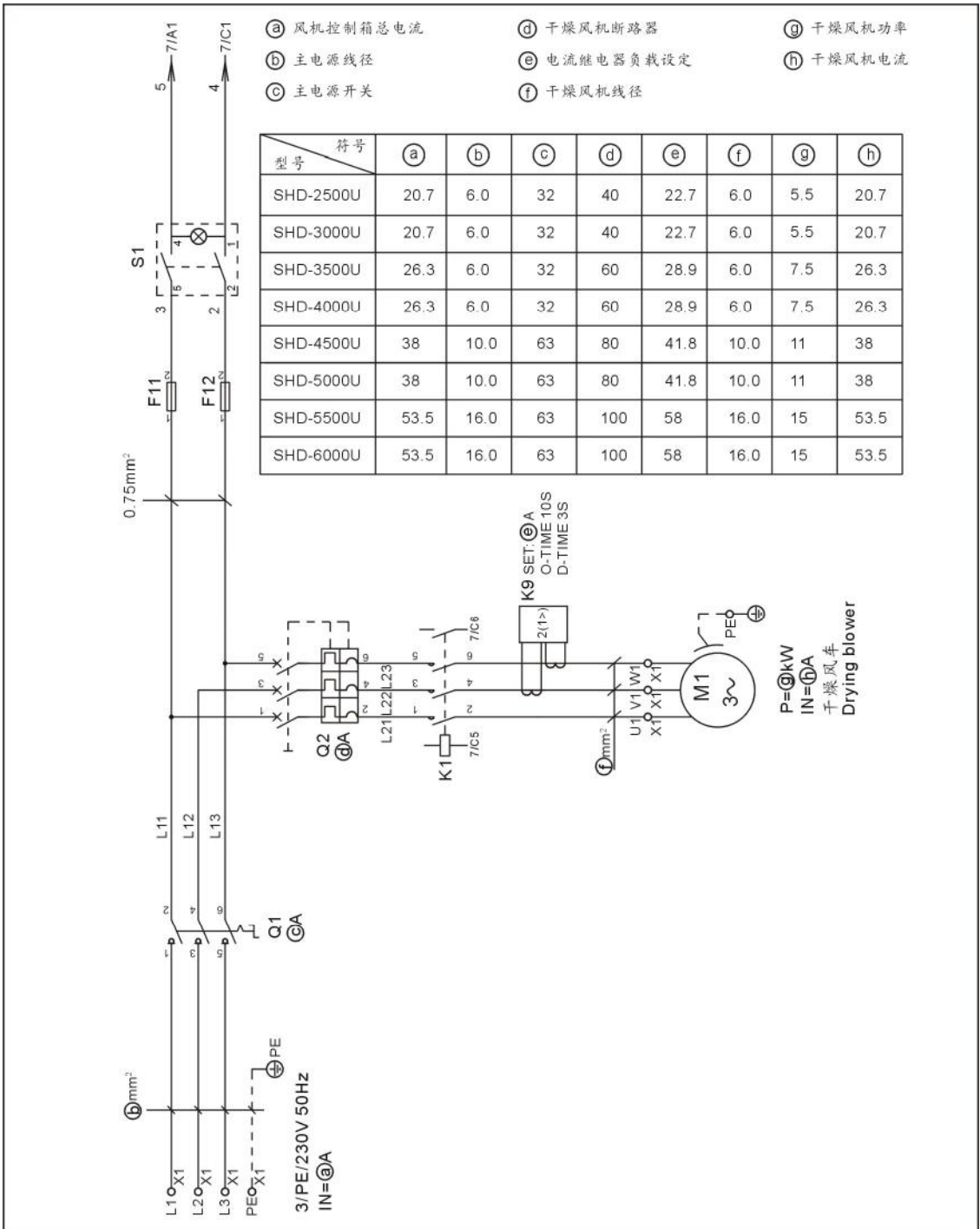
图 2-23: 主电路图一(SHD-2500U~6000U 230V)
