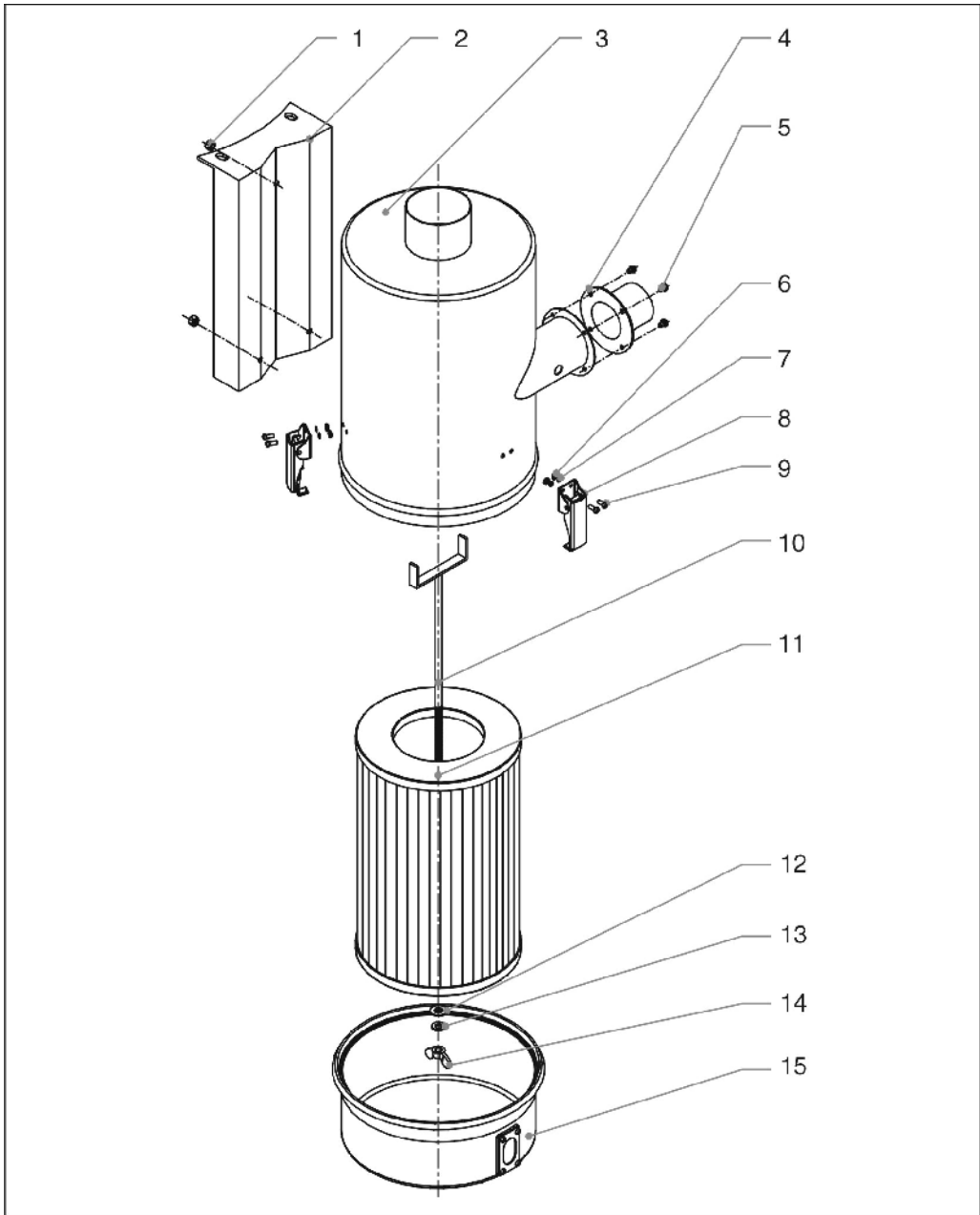
图 2-37: 欧化热风回收器分解图
