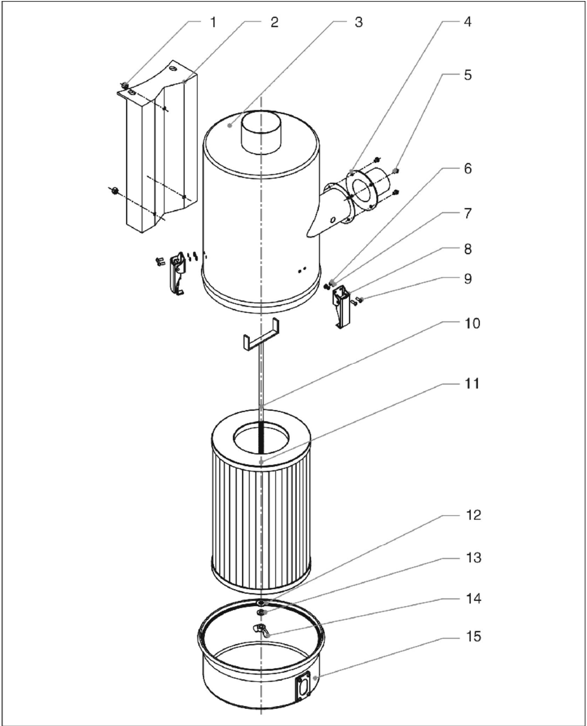
图 2-56: 欧化空气滤清图
