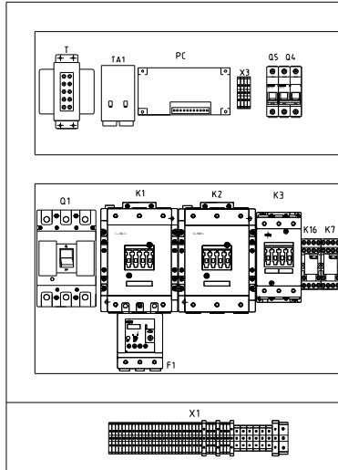
标准机型布局图
