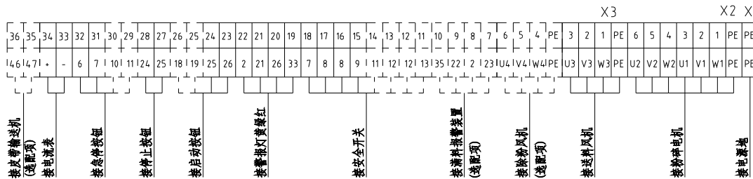
X10金属接头接线示意图 接满料报警装置 (选配项)
