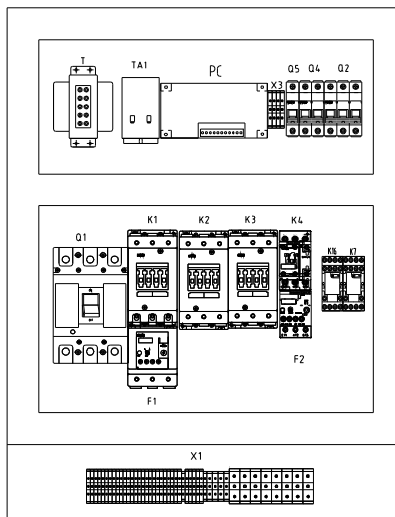
标准机型布局图
