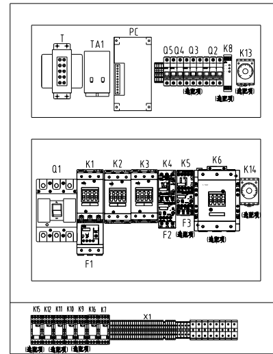
选配机型布局图
