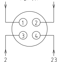
X10金属接头接线示意图 接满料报警装置 (选选项)
