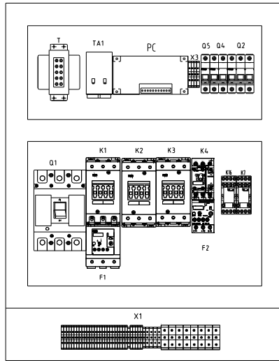
标准机型布局图
