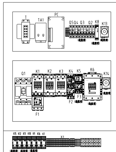
选配机型布局图
