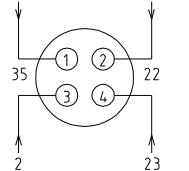
X10金属接头接线示意图 接清料报警装置 (选选项)
