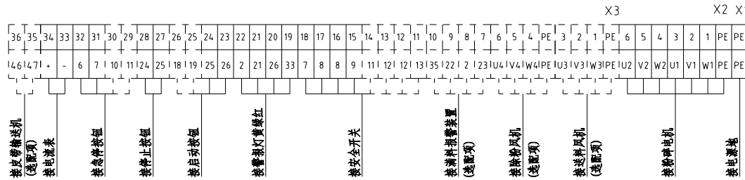
X10 金属接头接线示意图 接满料报警装置 (选选项)
