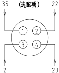
X10 金属接头接线示意图 接满料报警装置 (选选项)
