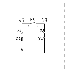
X4金属接头接线示意图 接皮带输送机 (选选项)
