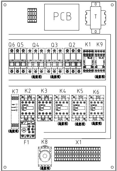
选装选配项装配图
