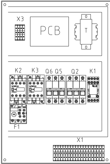
标准装配图
