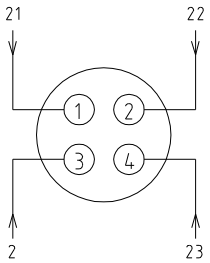
X10金属接头(选配项)
