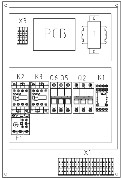
标准装配图
