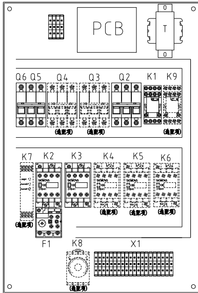
选装选项装配图
