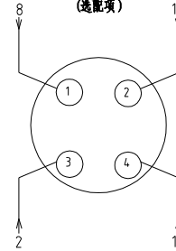
X10金属接头接线示意图 接满料报警装置 (选配项)
