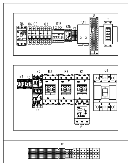
标准机型布局图
