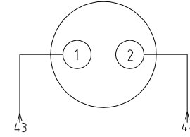
X7金属接头接线示意图 接皮带输送机 (选选项)
