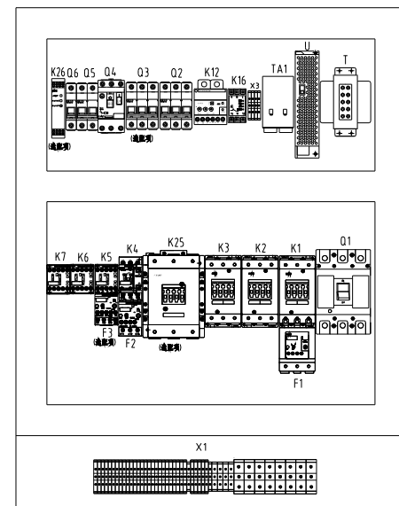
选配机型布局图
