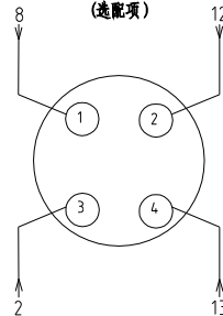
X10金属接头接线示意图 接满料报警装置 (选选项)
