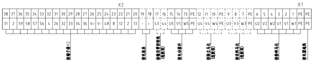
标准机型布局图
