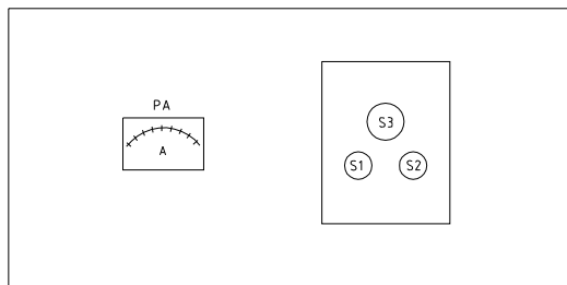
电控箱顶部
