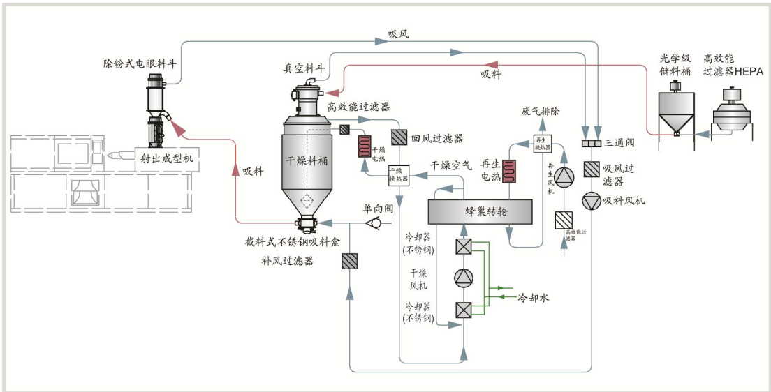
图 2-1: 工作原理示意图
