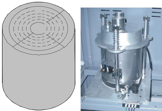
图 6-6: 蜂巢转轮图
