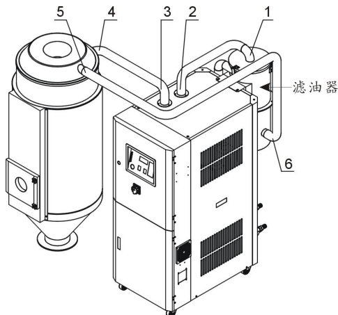
图 3-6: 滤油器安装图
