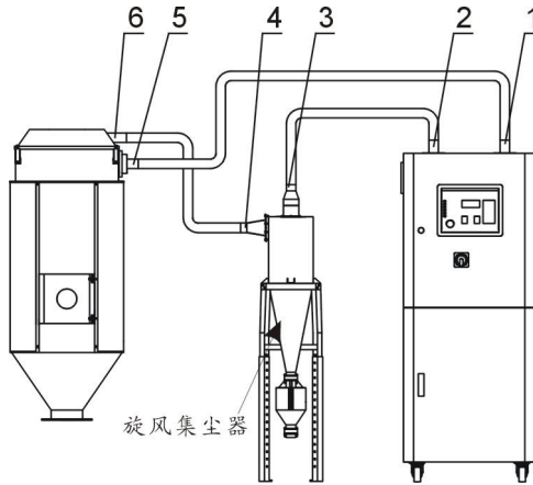
图 3-5: 旋风集尘器安装图
