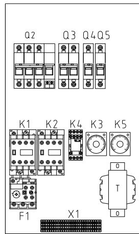
电控箱底板
