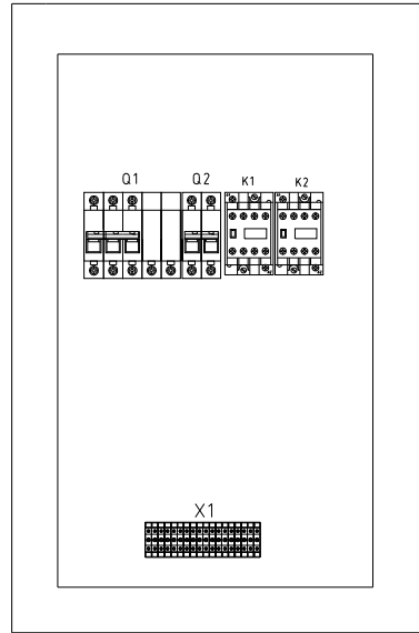
电箱底板 Base plate of electrical box
