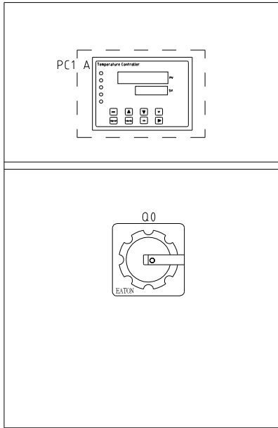
电箱面板 Electric box panel
