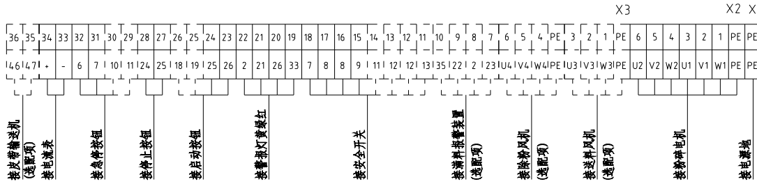
X10 金属接头接线示意图 接满料报警装置 (选配项)
