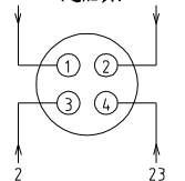
X10金属接头接线示意图 接满料报警装置 (选配项)
