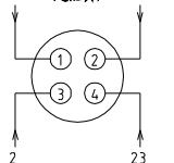
X10金属接头接线示意图 接满料报警装置 (选配项)
