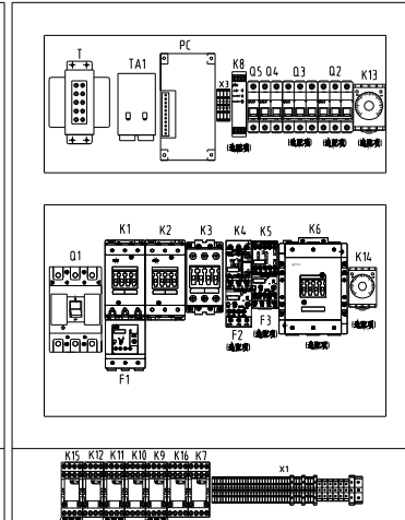
选配机型布局图
