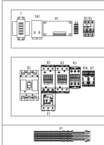
标准机型布局图
