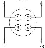
×10 金属接头接线示意图 接满料报警装置 (选选项)
