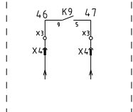
选配皮带输送机控制触点接线示意图
