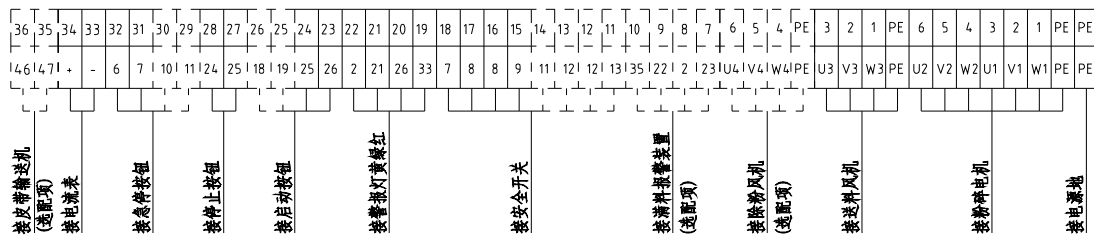
X10金属接头接线示意图 接满料报警装置 (选配项)
