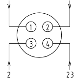
X10 金属接头接线示意图 接满料报警装置 (选配项)
