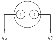
X4 金属接头接线示意图 接皮带输送机 (选配项)
