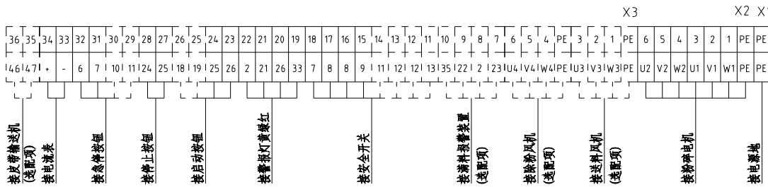
×10 金属接头接线示意图 接满料报警装置 (选选项)
