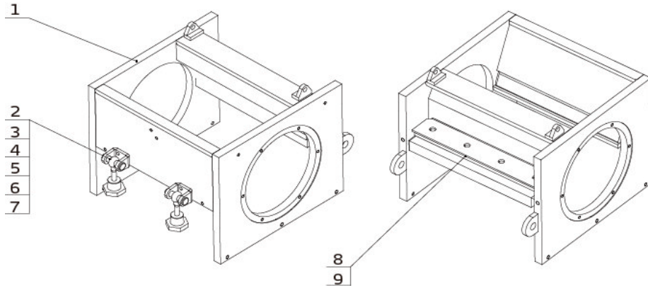
图 3-1: 粉碎室总成一
