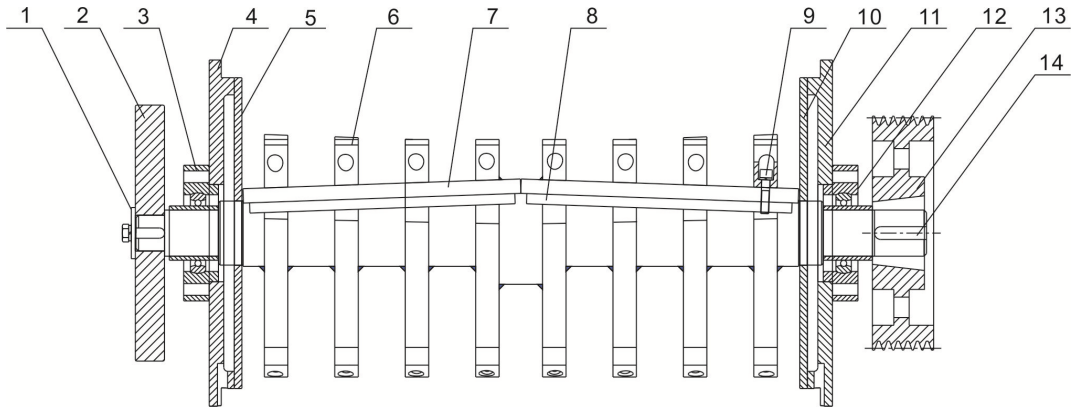
图 5-1: 粉碎室总成三图(SG-60110EB)
