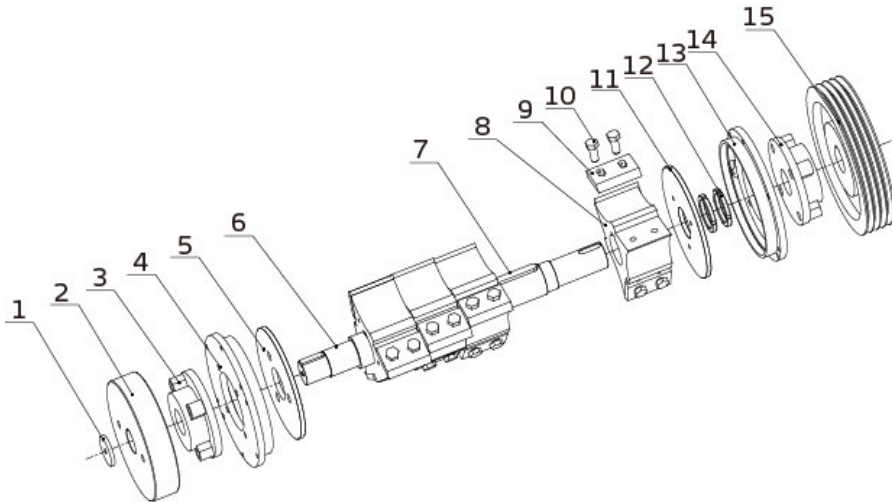
图 4-1：粉碎室总成二图
