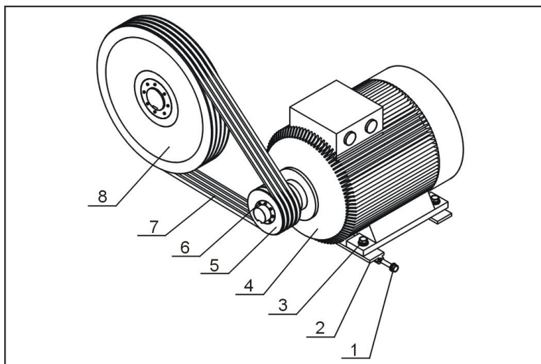
图 2-1：主传动装置图
