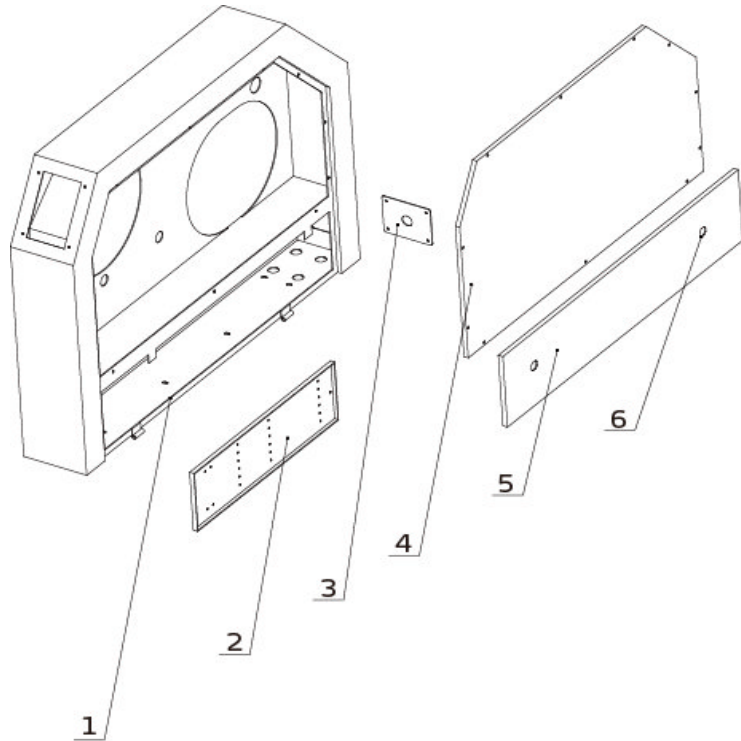
图 7-1：护罩部件图
