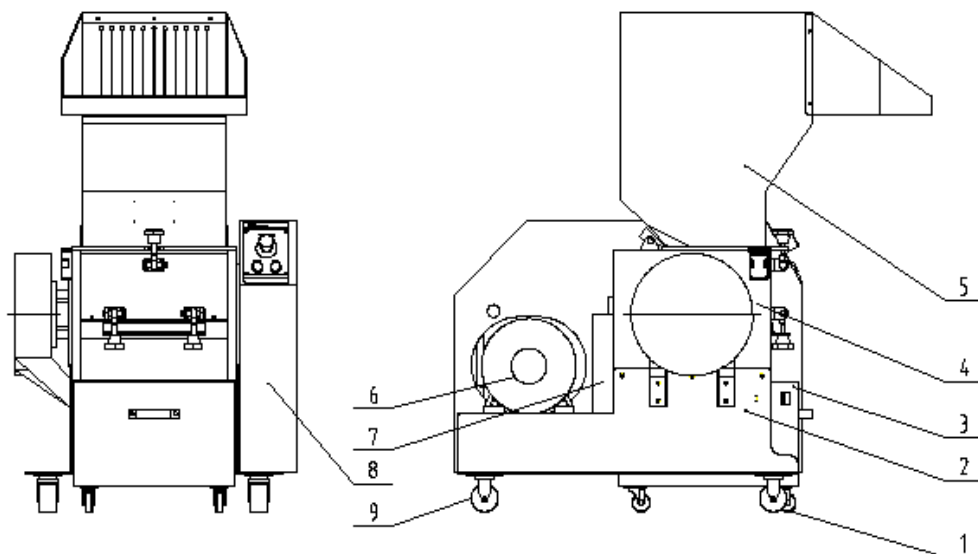
图 1-1：系统结构图
