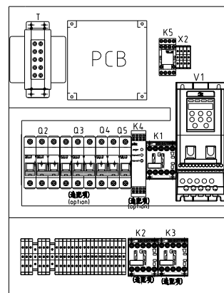
选配机型布局图 Optional Model Layout
