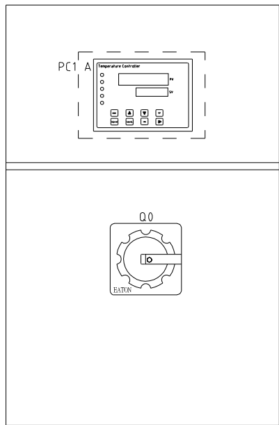
电箱面板
