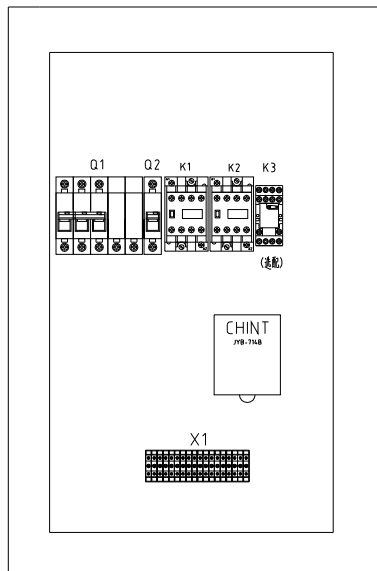
电箱底板
