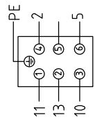
X3(料斗与主机互连重载接头)
