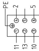
X3(料斗与主机互锁重负载头)
