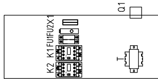
SHD-100SL-200SL 电气布置图
