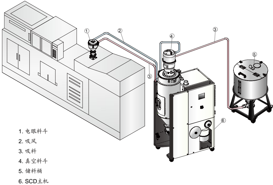
图 3-2: 安装示意图(全封闭式)
