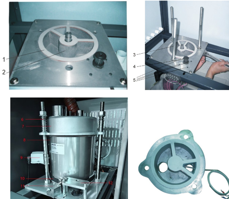
图 6-7: 蜂巢转轮安装示意图
