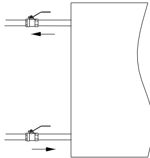
图 3-4: 冷却水连接示意图
