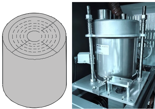
图 6-6: 蜂巢转轮图
