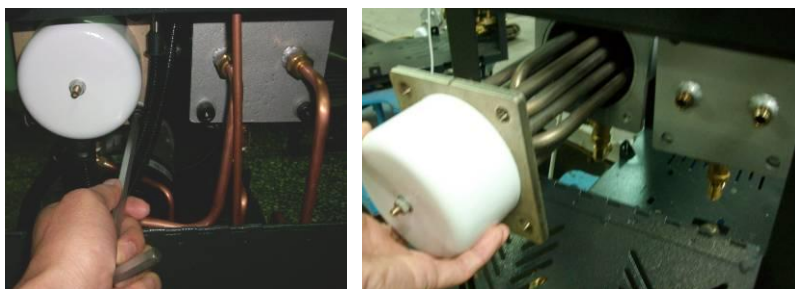
图 6-7: 电热管二
