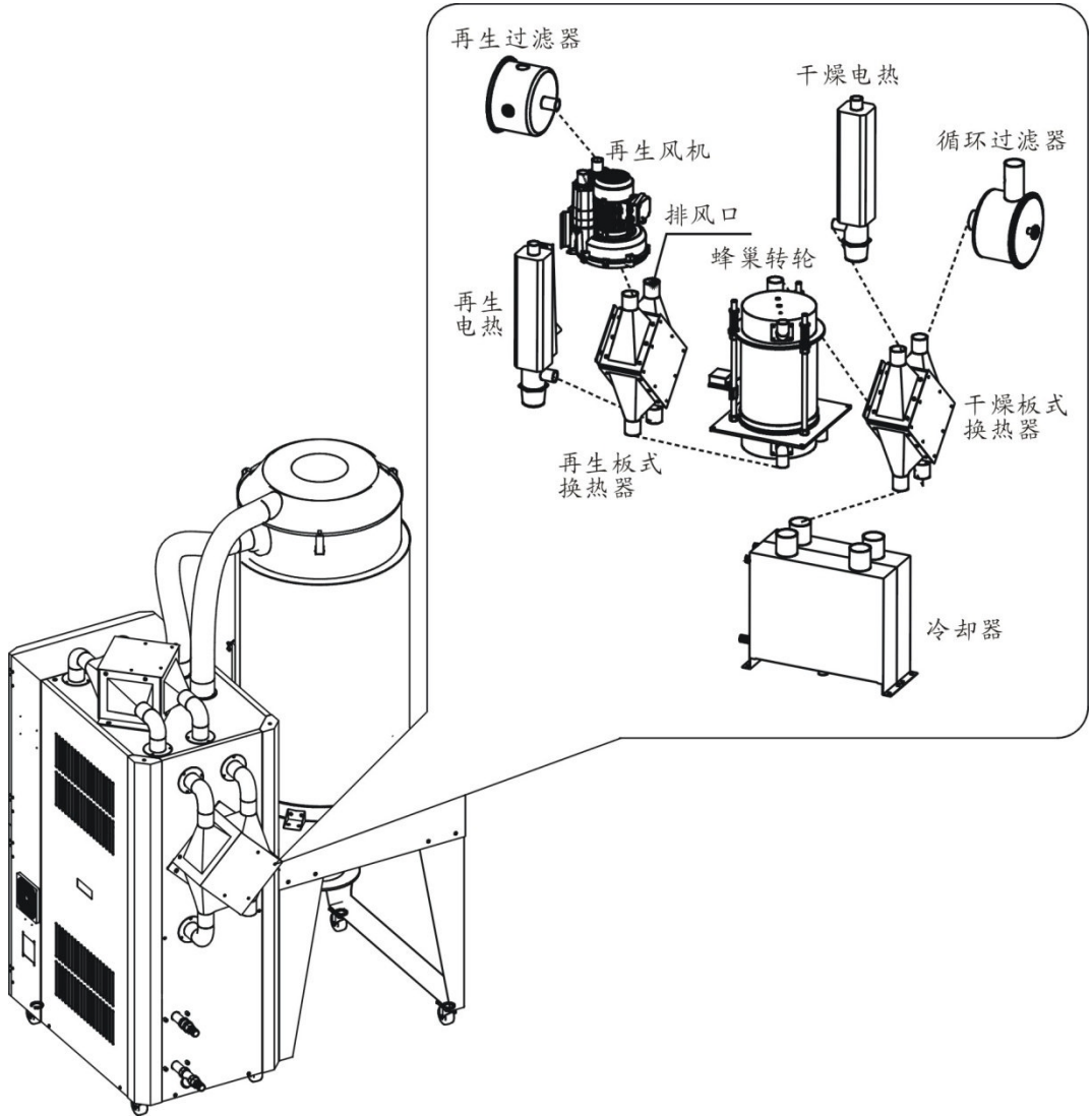
图 3-5: 板式换热器接管图
