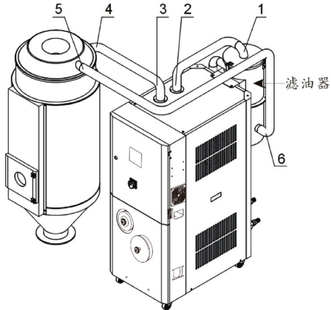
图 3-4：滤油器安装图
