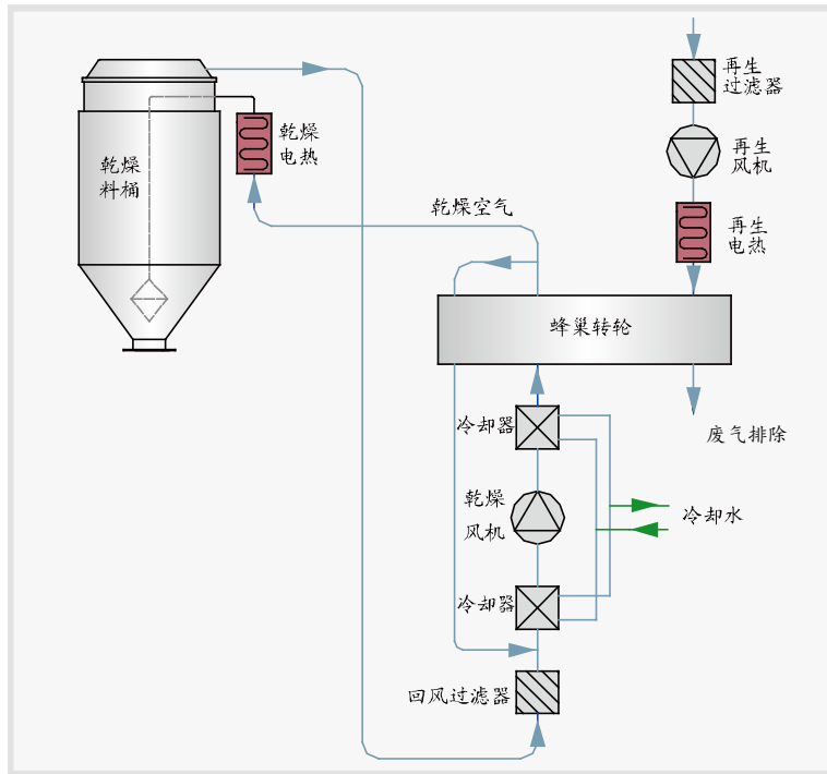
图 2-1: 工作原理示意图
