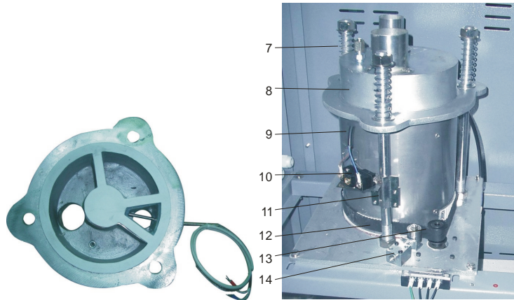
图 6-3: 蜂巢转轮安装示意图
