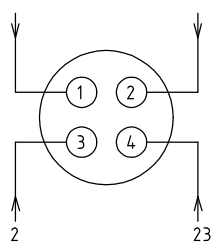
X10 金属接头接线示意图 (选选项)
