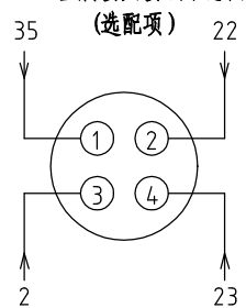
X10 金属接头接线示意图
