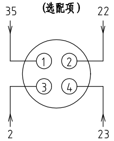
X10 金属接头接线示意图 (选配项)
