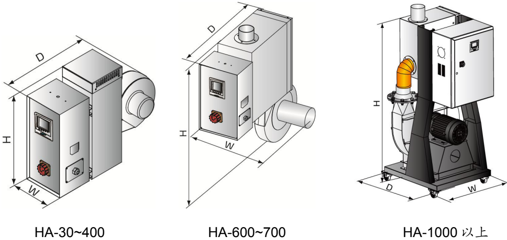
图 1-1: 外形尺寸图
