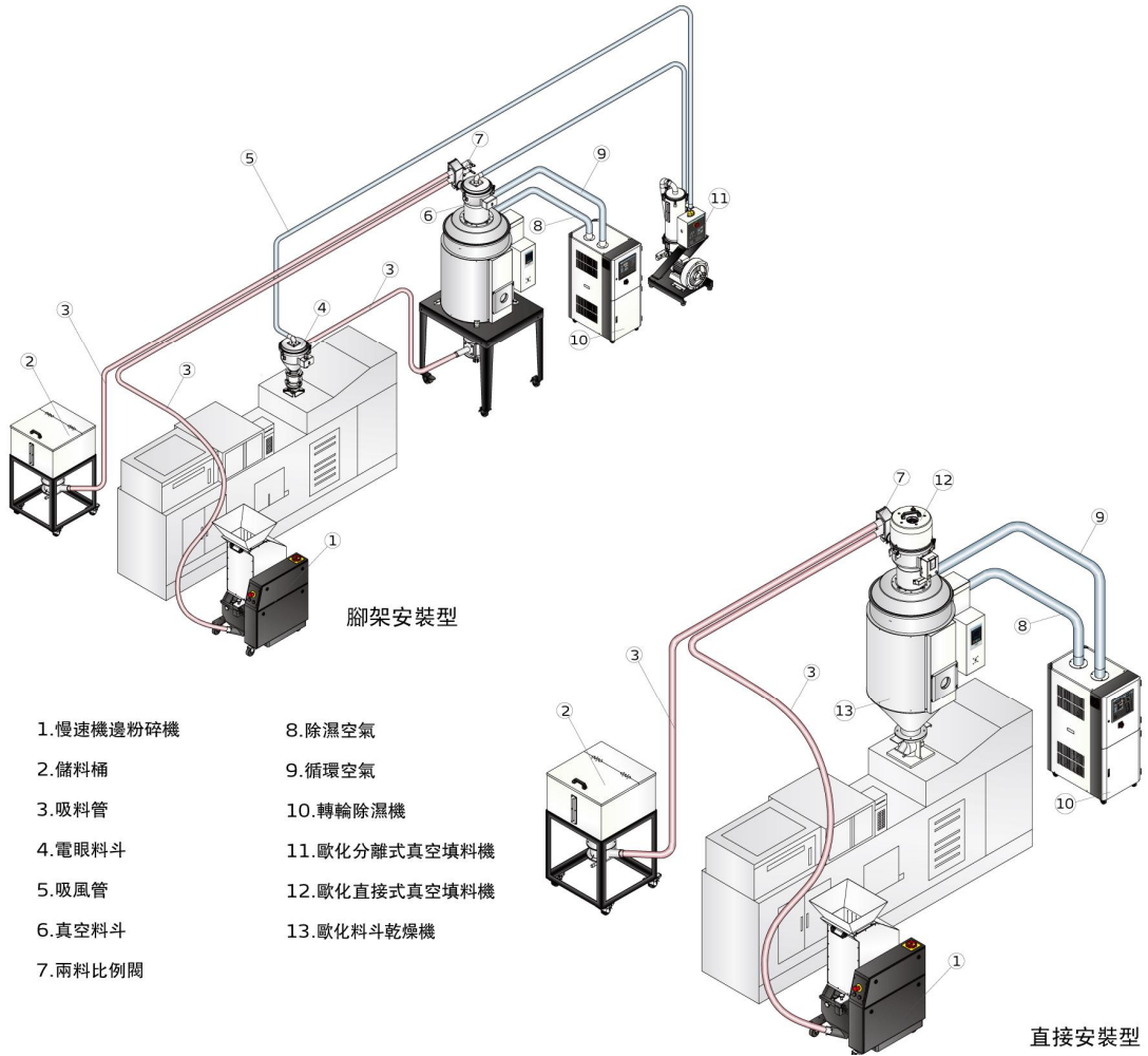
图 2-2: 注塑机上安装示意图
