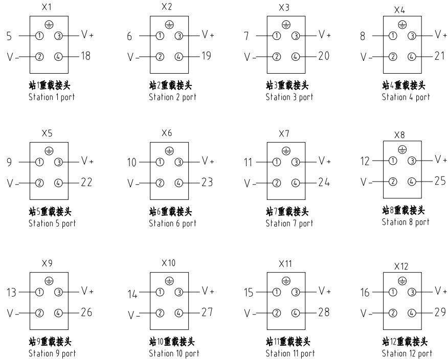
注：4P重载接头定义
