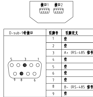
SCAL 5HP RS-485接口定义
