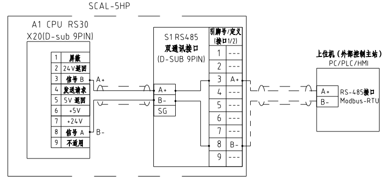
SCAL RS-485通讯接线示意图
