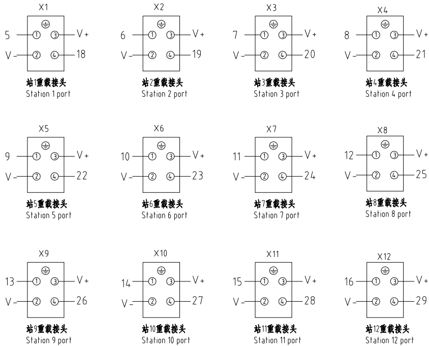
注：4P重载接头定义
