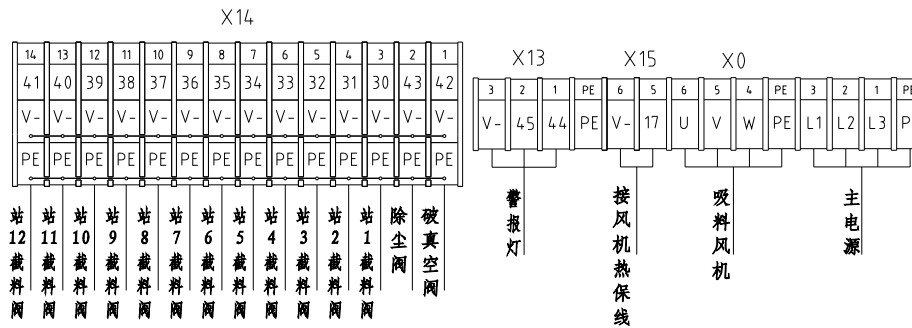
电气底板
