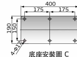
底座安裝圖 C
